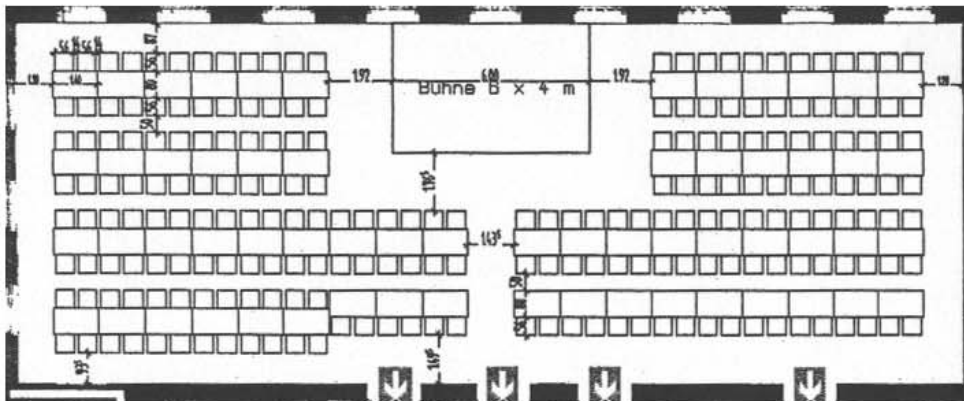
Tischbestuhlung für 216 Personen mit Bühne 6x4m
